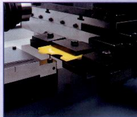
Dima e tastatore Template and stylus Gabarit et doigt de copiage Schablone und Taster
