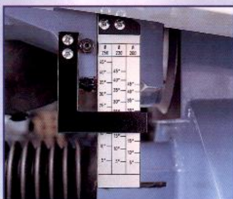
Scala di riferimento per spoglia posteriore Back clearance reference scale Echale de référence pour la dépeuille postérieur Masstab für Winkel hinten
